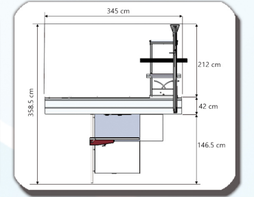
ÇİZİCİLİ YATAR DAİRE 3200 YERLEŞİM PLANI CIRCULAR SAW 3200 LAYOUT PLAN
