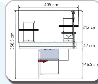
ÇİZİCİLİ YATAR DAİRE 3800 YERLEŞİM PLANI CIRCULAR SAW 3800 LAYOUT PLAN
